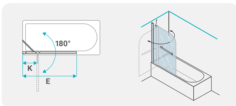
Parete per vasca con elemento fisso / bath tub wall fix side / paroi baignoire partie fixe / badewannenwand festseite / pared bañera lado fijo
