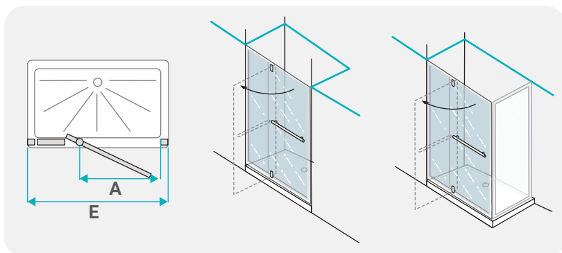
Porta battente con elemento fisso / pivot door with fix side / porte tournante avec paroi / flügeltür mit festseite / puera batiente pared fija
